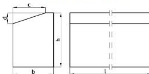
Rys. 2. Wymiarowanie krawężników
