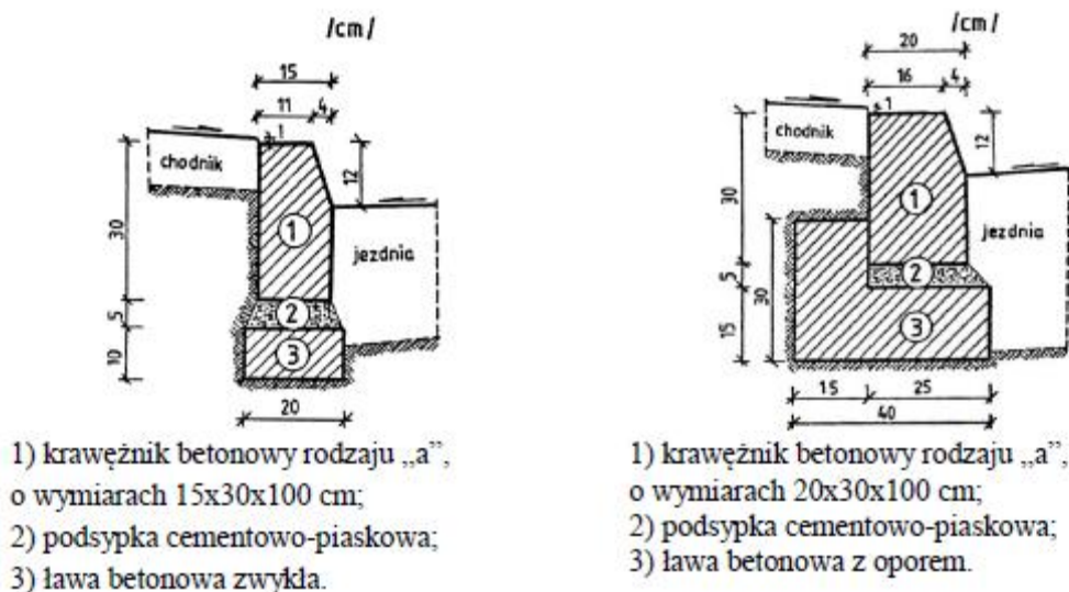
Rys. 3. Przykładowe ustawienie krawężników na ławie betonowej
