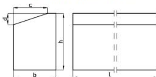
Rys. 2. Wymiarowanie krawężników
