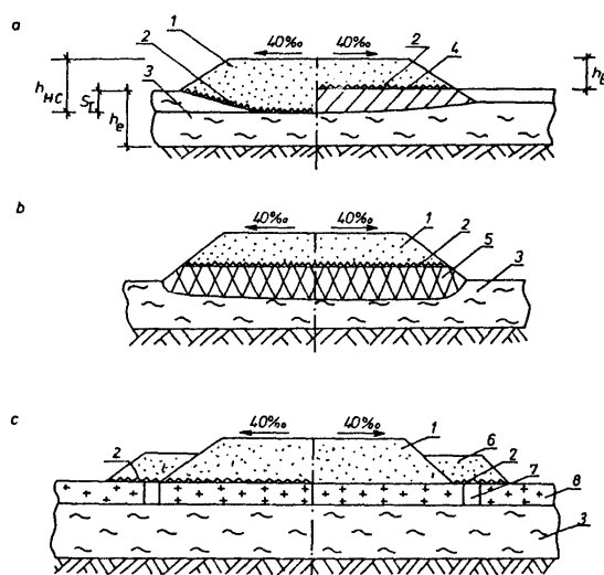
Rys. 3.1. Konstrukcje dróg tymczasowych na gruntach słabonośnych
