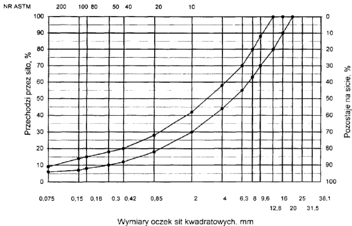
Rys. 6. Krzywe graniczne uziarnienia mieszanki mineralnej AC16S
