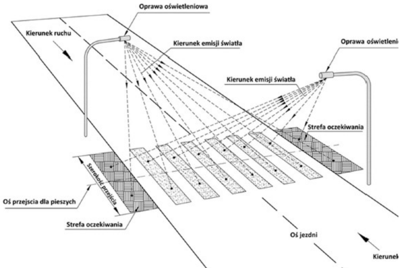
Schemat rozmieszczenia opraw oświetleniowych przed przejściem dla pieszych.
