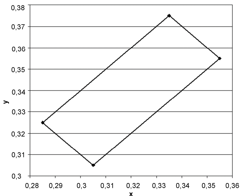
Rys. 1. Współrzędne chromaticzności x, y dla barwy białej oznakowania.
