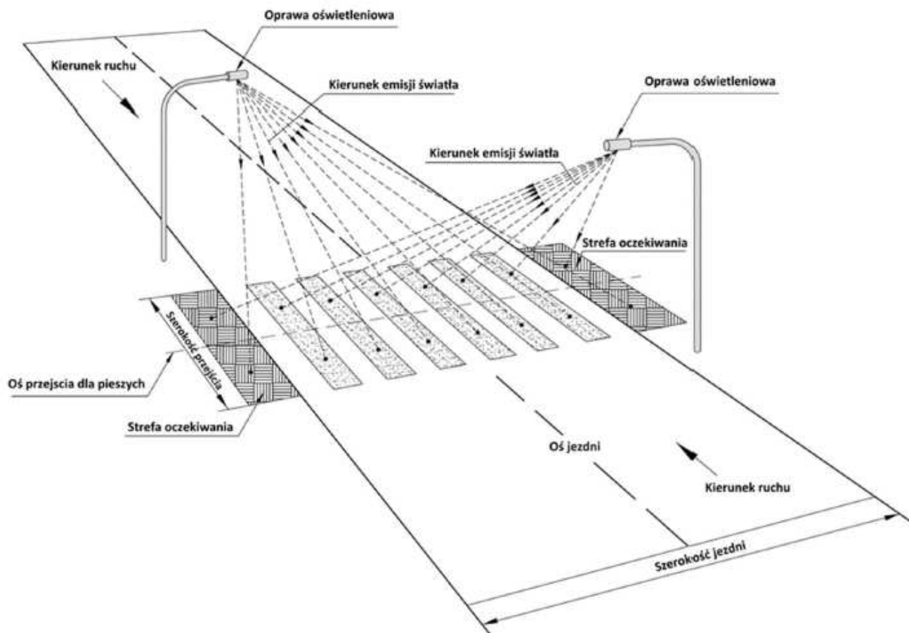
Schemat rozmieszczenia opraw oświetleniowych przed przejściem dla pieszych.
